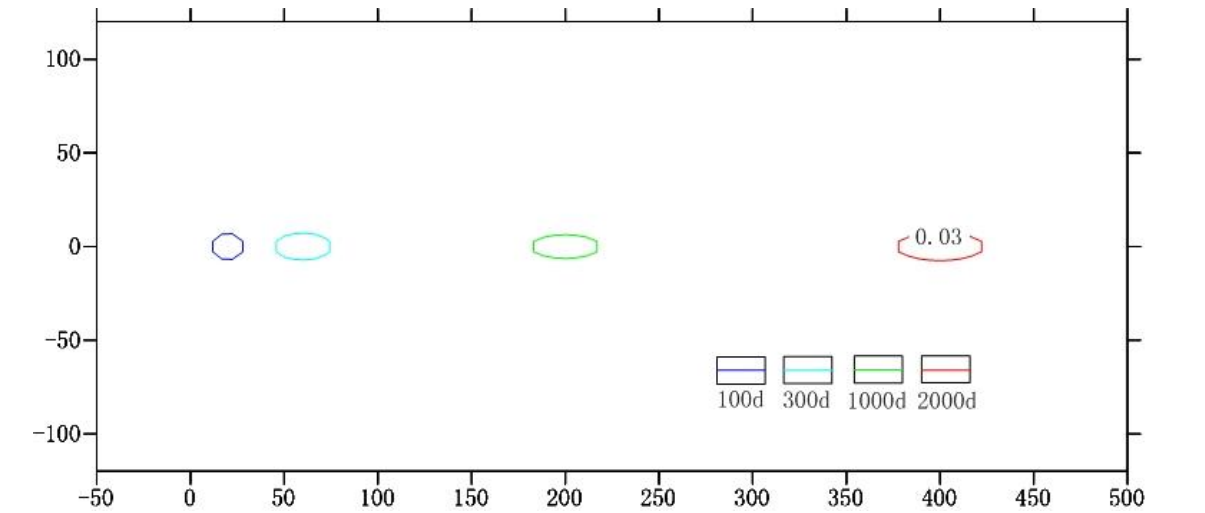
图 6 汽油储罐管道泄漏污染物在浅层含水层中运移图
